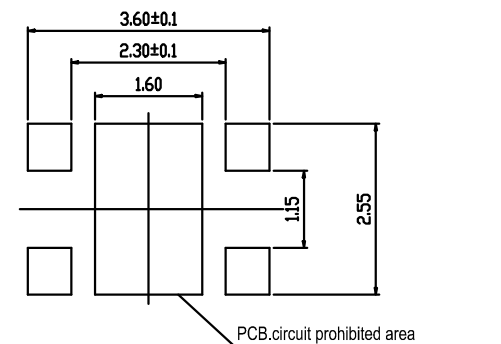
开关示意图
